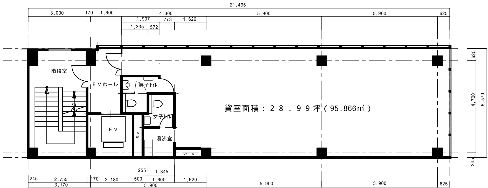
3 ~ 5 階 ( 基準階 ) 平面図
